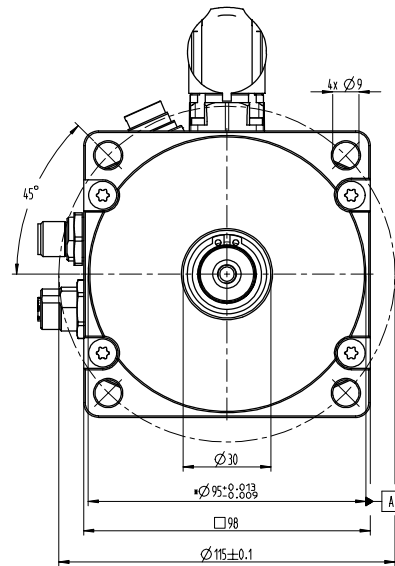
Flange version for assembly from the rear side/ Flangeversion für Montage von hinten
