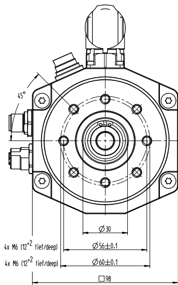
Flange version for assembly from the front/ Flangeversion für Montage von vorne
